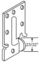
900-17778 Roller Bracket
