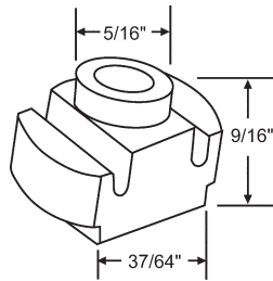
900-9936 Drawer guide
