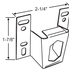
900-11843
