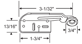
45-25
