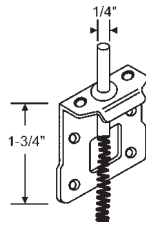
2-68 Top Pivot
