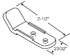
900-847 Door Aligner
