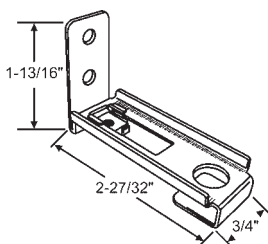
7-278 Pivot L-Bracket
