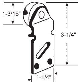
3-193 1/16" Offset
