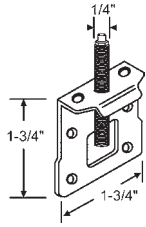
2-69 Bottom Pivot
