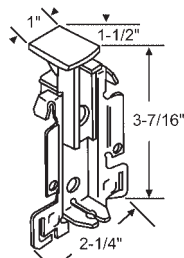
900-12459 Top Guide
