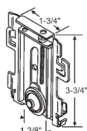
900-11827 Bottom Roller
